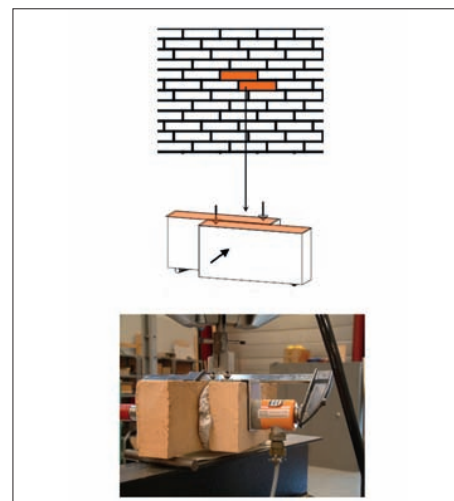
Figur 2. Princippet i SBI's vridningsprøvning. Under prøvningen er der med en skruetvinge påført et tryk på tværs, som skal efterligne trykket fra det ovenfor liggende murværk
