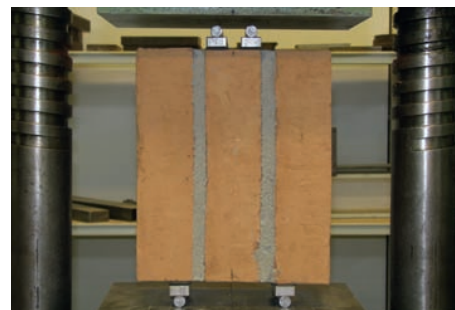
Figur 1. Teglstensprøvelegeme i henhold til DS/EN 1052-3
