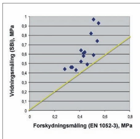
Figur 3. Sammenligning af forskydningsstyrke målt ved trestensprøvning og ved vridningsmetoden. Forsøget er udført på 5 typer mørtel KC50/50/750 kombineret med 3 typer mursten. Hvert punkt er midelværdi af 6 prøvninger
