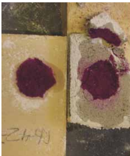
Figur 9. Karbonatiseringsdybde i prøverne blev målt efter brud ved påsprøjtningen af indikatoren phenolphthalein
