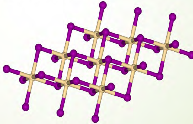
\text{CaOH}_2 Kalciumhydroxid
